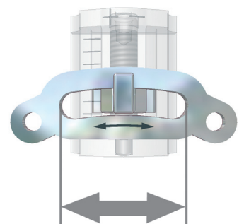
Große, laterale Beweglichkeit von 17°/7,5 mm
