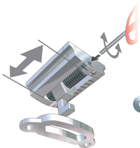
Großer, sagittaler Verstellweg von 7 mm
